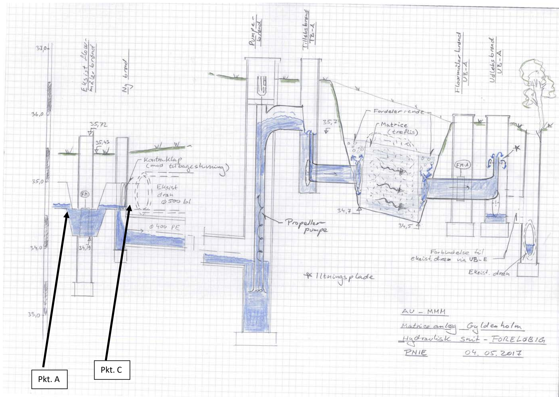
Fig 6. Eksisterende flowmåler brønd (Pkt. A, til venstre) Flowdeler brønd, pkt. C. Design af MMM bassin og installationer (til højre).
