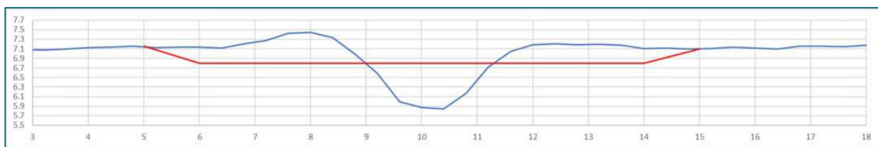
Figur 2. Eksempel på tværsnit af terrænmodel (blå streg) og skitsering af terrænafgnavningen (rød streg). Figuren er anvendt i Teknisk forundersøgelse for Lavbundsprojekt i Ringfener (Naturstyrelsen/COWI, 2021)
