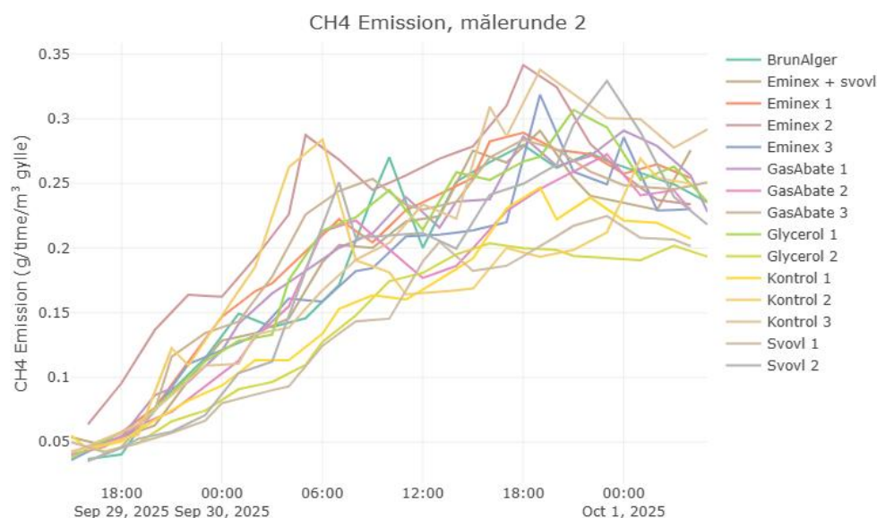
Figur 7: Koncentrationer af metan emission pr. flaske for kontrolrunde. I kontrolrunden var der ikke tilsat additiver i flaskerne, og dermed ses den naturligt forekommende variation fra indholdet i flaskerne. Navngivningen af graferne er på baggrund af tildelingen af additiver i målerunde 3.
