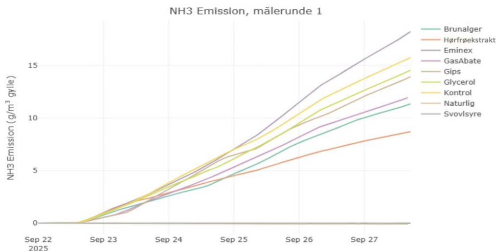
Figur 6. Kumulative ammoniakemissioner over tid for de forskellige behandlinger i målerunde 1. Kontrollen repræsenterer ubehandlet gylle, og tidsangivelsen viser den tid, der er gået efter tilsætning af additiver.
