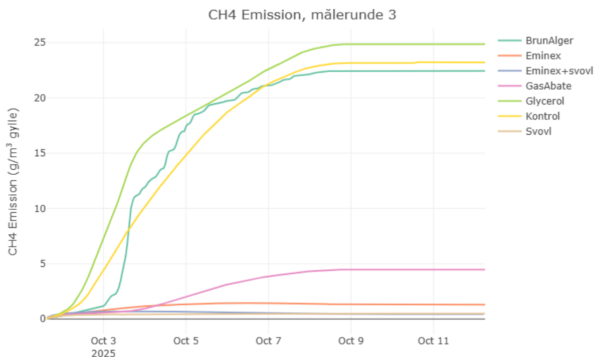
Figur 9: Metanemission pr. behandling (gennemsnit af replikationer) i g/time/m 3 gylle i målerunde 3. Kontrollen repræsenterer ubehandlet gylle, og tidsangivelsen viser den tid, der er gået efter tilsætning af additiver.
