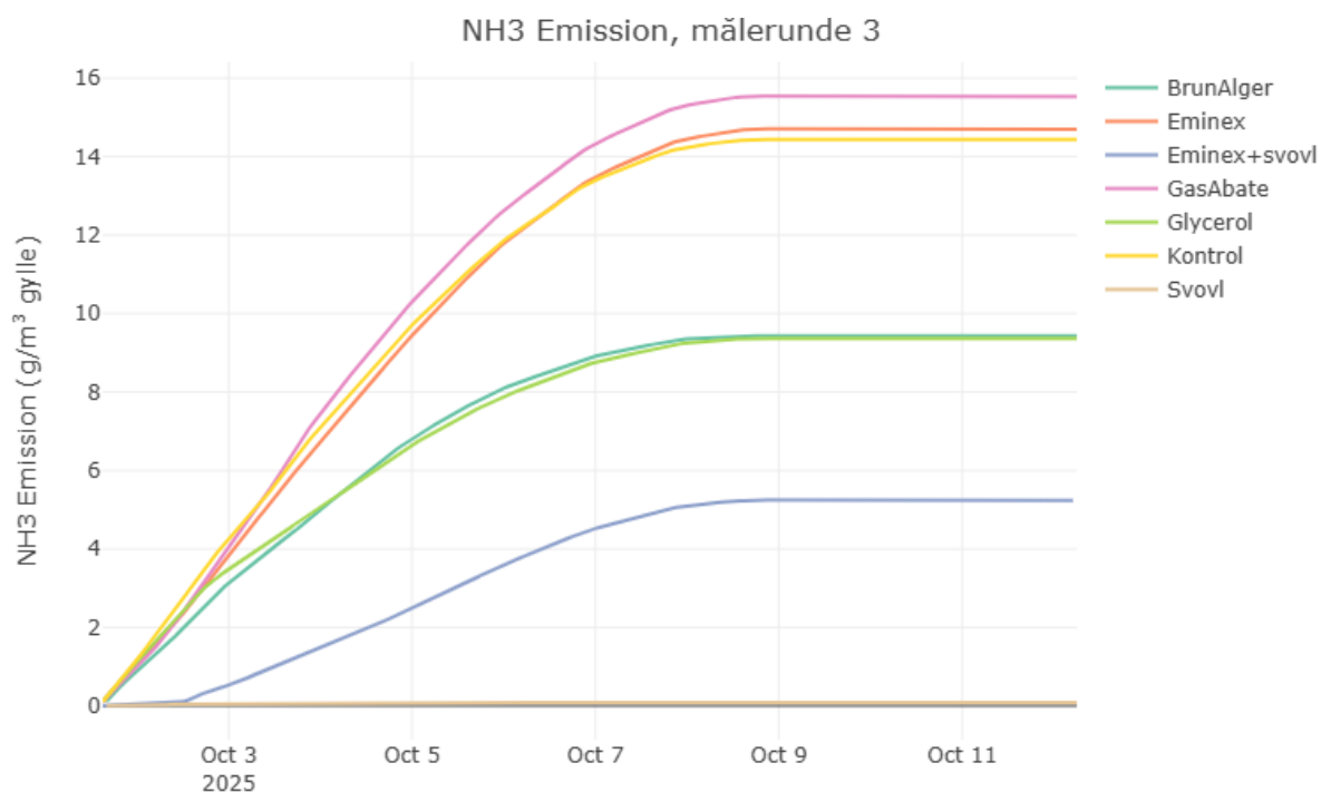
Figur 11: Ammoniakemission pr. behandling (gennemsnit af replikationer) i g/time/m 3 gylle i målerunde 3. Kontrollen repræsenterer ubehandlet gylle, og tidsangivelsen viser den tid, der er gået efter tilsætning af additiver.
