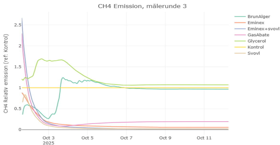
Figur 3: Relativt kumulative metanemissioner over tid for de forskellige behandlinger i målerunde 3. Kontrollen repræsenterer ubehandlet gylle (negativ kontrol) og er referencen for behandlingerne sat til at være 1. Tidsangivelsen viser den tid, der er gået efter tilsætning af additiver d. 1. oktober 2025.
