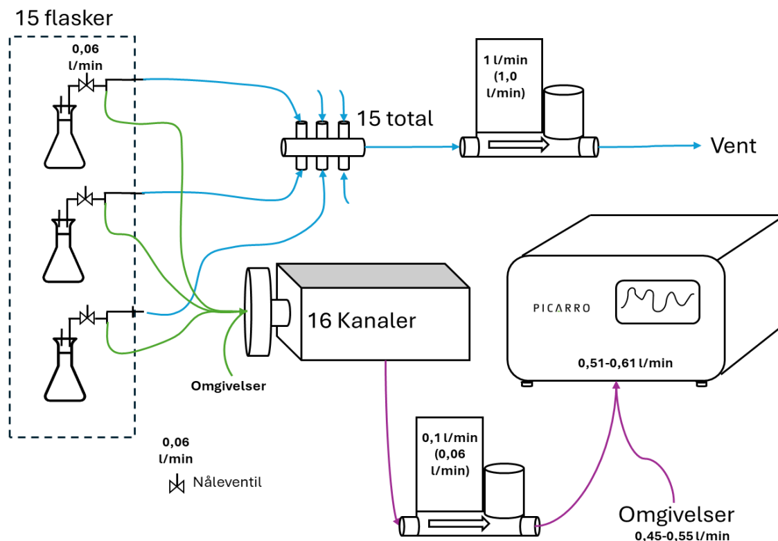
Figur 1: Koncept-skitse af forsøgsopstillingen, bestående af 15 Duran-flasker (2 l.) koblet til et lukket luftflowsystem. Luftstrømmen blev reguleret ved hjælp af MFC, og udlædningsluften blev pumpet til en Picarro G2509-analysator til kontinuerlig måling af drivhusgaskoncentrationer og ammoniak.
