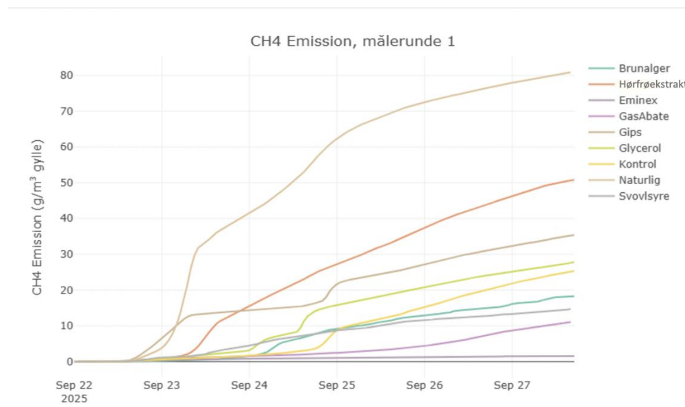
Figur 5: Kumulative metanemissioner over tid for de forskellige behandlinger i målerunde 1. Kontrollen repræsenterer ubehandlet gylle, og tidsangivelsen viser den tid, der er gået efter tilsætning af additiver.
