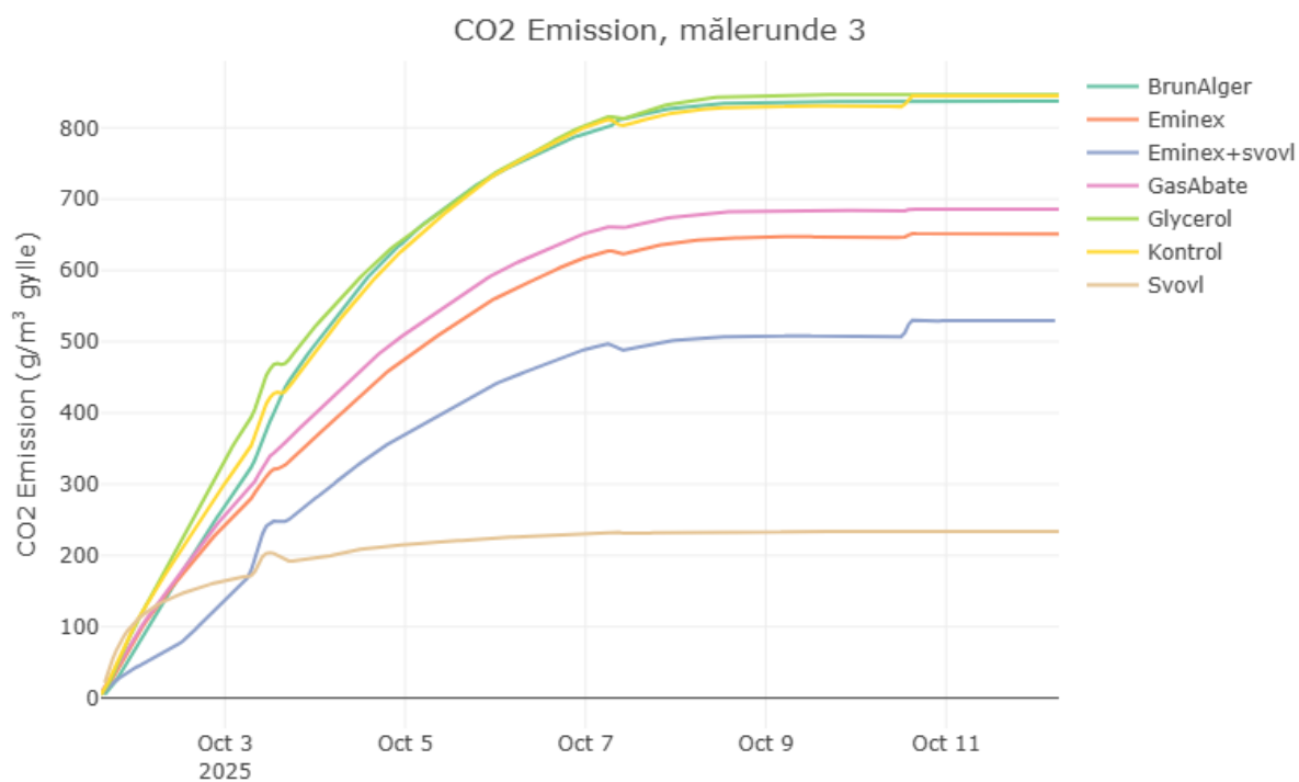
Figur 10: Kuldioxidemission pr. behandling (gennemsnit af replikationer) i g/time/m 3 gylle i målerunde 3. Kontrollen repræsenterer ubehandlet gylle, og tidsangivelsen viser den tid, der er gået efter tilsætning af additiver.
