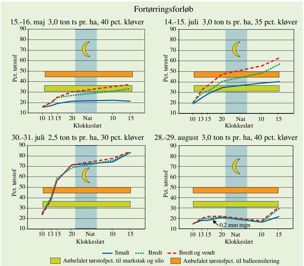
Figur 3. Tørstofprocenten gennem fire forskellige fortørringsforløb for rødkløvergræs. Der er høstet kl. 10, og tørstofprocenten er fulgt indtil kl. 15 næste dag.
