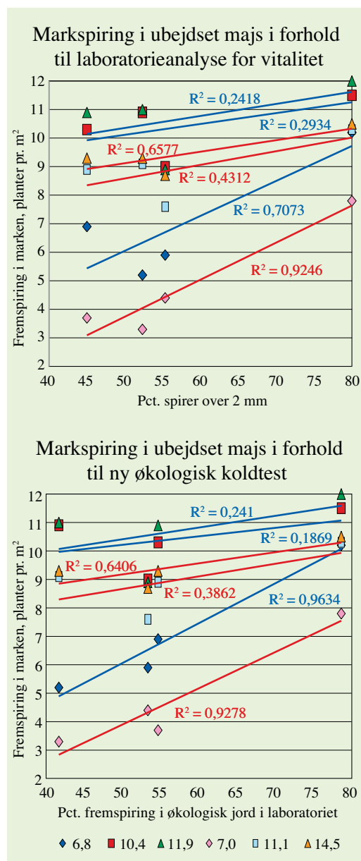
Figur 5. Sammenhæng mellem spiring i papirruller og markspiring (øverst) og koldtest i økologisk jord og markspiring (nederst). Majs er sået på to lokaliteter på tre forskellige såtider. Hver linje illustrerer en såtid på en lokalitet. Jo tættere R 2 værdien er på 1, jo bedre er sammenhængen mellem laboratorieanalyse og markspiring. Signaturforklaringen er jordtemperaturen ved såning.
