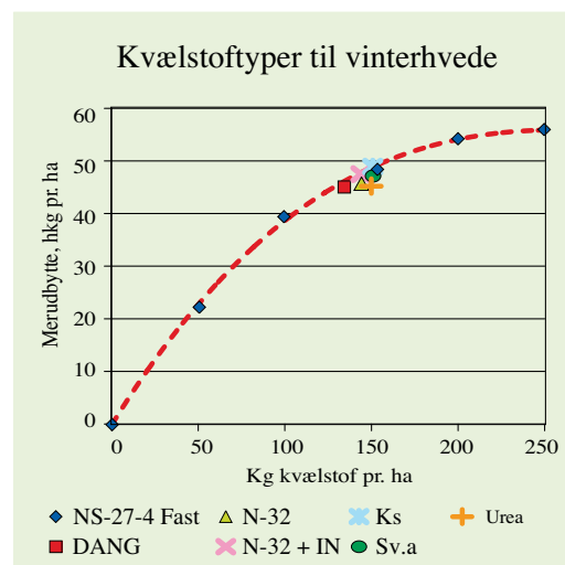
Figur 9. Merudbytte for tilførsel af forskellige kvælstoftyper til vinterhvede.
