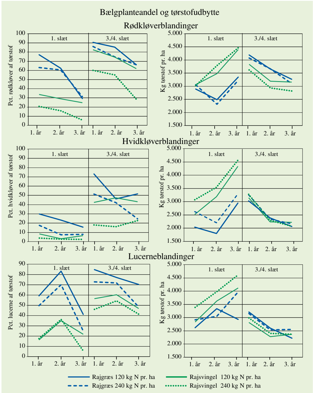
Figur 1. Bælglanteandel i procent af afgrødetørstof og udbytte ved første slæt og i tredje eller fjerde slæt (august slæt) i første til tredje brugsår (2006 til 2008). Alle parceller er høstet på samme dag. Sorter: Rødkløver (Rajah), hvidkløver (Milo), lucerne (Pondus), alm. rajgræs (Mikado) og rajsvingel (Perun).
