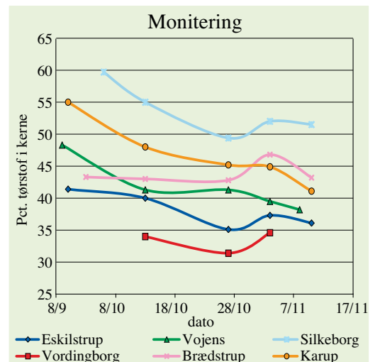
Figur 6. Monitering af vandprocenten i kernemajs i seks marker i tiden op til høst.
