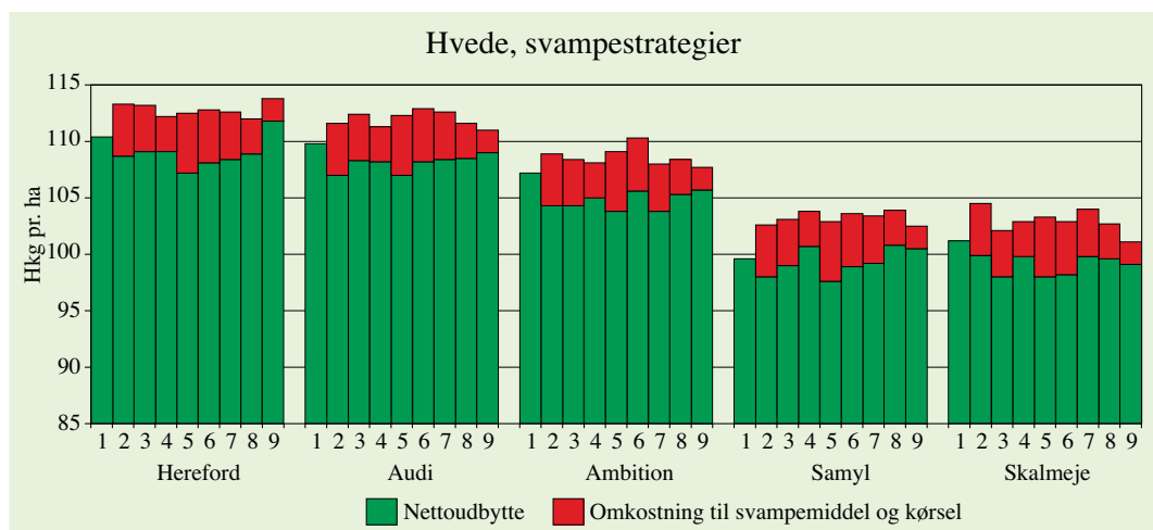
Figur 12. Opnåede brutto- og nettonetudbytter for forskellige svampestrategier i de fire forsøg i tabel 36. De respektive forsøgsled er markeret under søjlerne.
