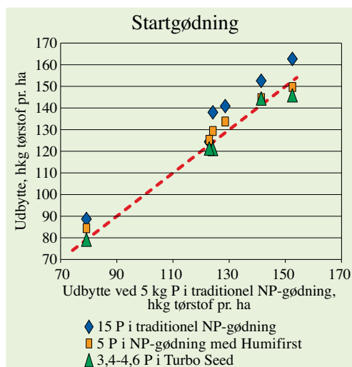
Figur 4. Udbyttet i seks forsøg i 2007 og 2008 ved placering af 15 kg fosfor pr. ha i en traditionel NP-gødning, 5 kg fosfor pr. ha i en Humifirst-baseret NP-gødning og 3,4 til 4,6 kg fosfor pr. ha i mikrogranulatgødningen Turbo Seed i forhold til placering af 5 kg fosfor pr. ha i en traditionel NP-gødning. Turbo Seed har været med i fem forsøg, heraf Turbo Seed med Humifirst i to forsøg og uden Humifirst i tre forsøg. Turbo Seed er placeret direkte i såsporet. De øvrige NP-gødninger er placeret 5 cm ved siden af og 5 cm under frøene. Den stiplede linje markerer udbyttet ved placering af 5 kg fosfor i traditionel startgødning.
