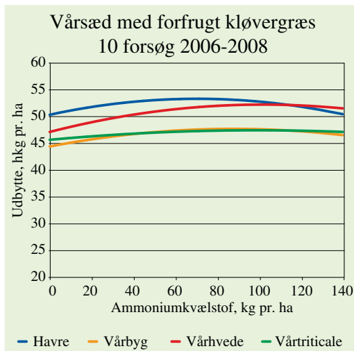
Figur 2. Responskurver for tilførsel af ammoniumkvælstof til havre, vårbyg, vårhvede og vårtriticale med forfrugt kløvergræs.
