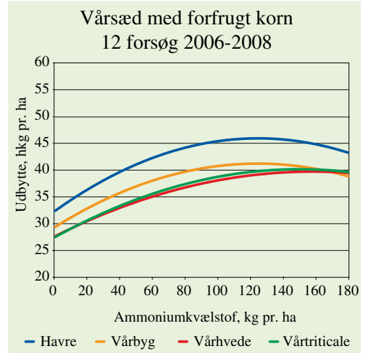
Figur 3. Responskurver for tilførsel af ammoniumkvælstof til havre, vårbyg, vårhvede og vårtriticale med forfrugt korn.
