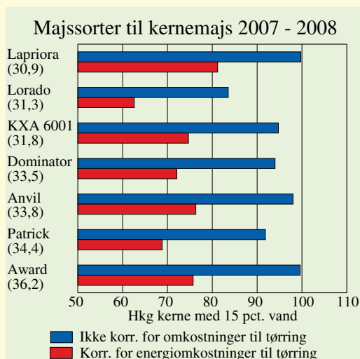
Figur 2. Majssorter til kernemajs 2007 og 2008. Gennemsnitsudbytte af hkg kerne pr. ha både med og uden korrektion for energiomkostninger til tørring. Tallet i parentes efter sortsnavnet er vandprocenten i kernerne ved høst.
