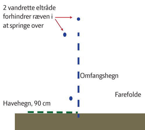
Figur 1.1 Eksempel på opbygning af rævesikret hegegn
