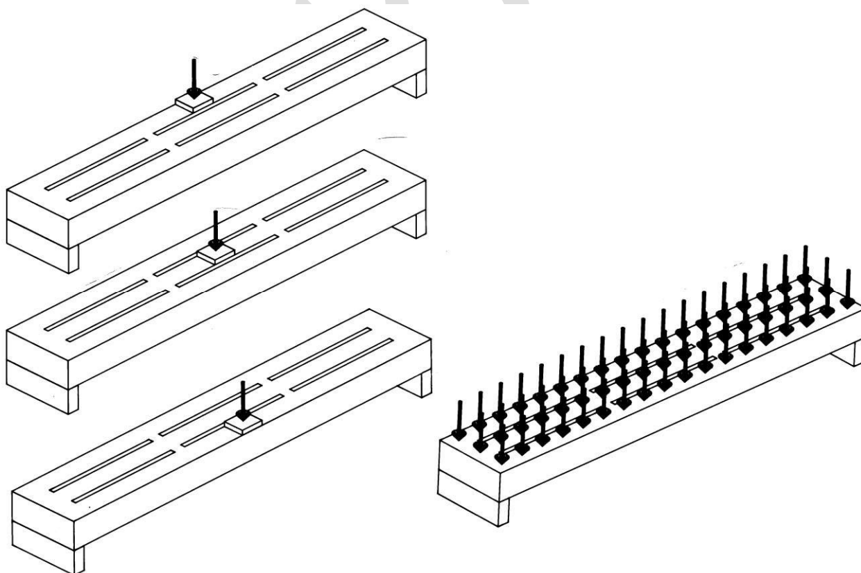
Punktlast Q
