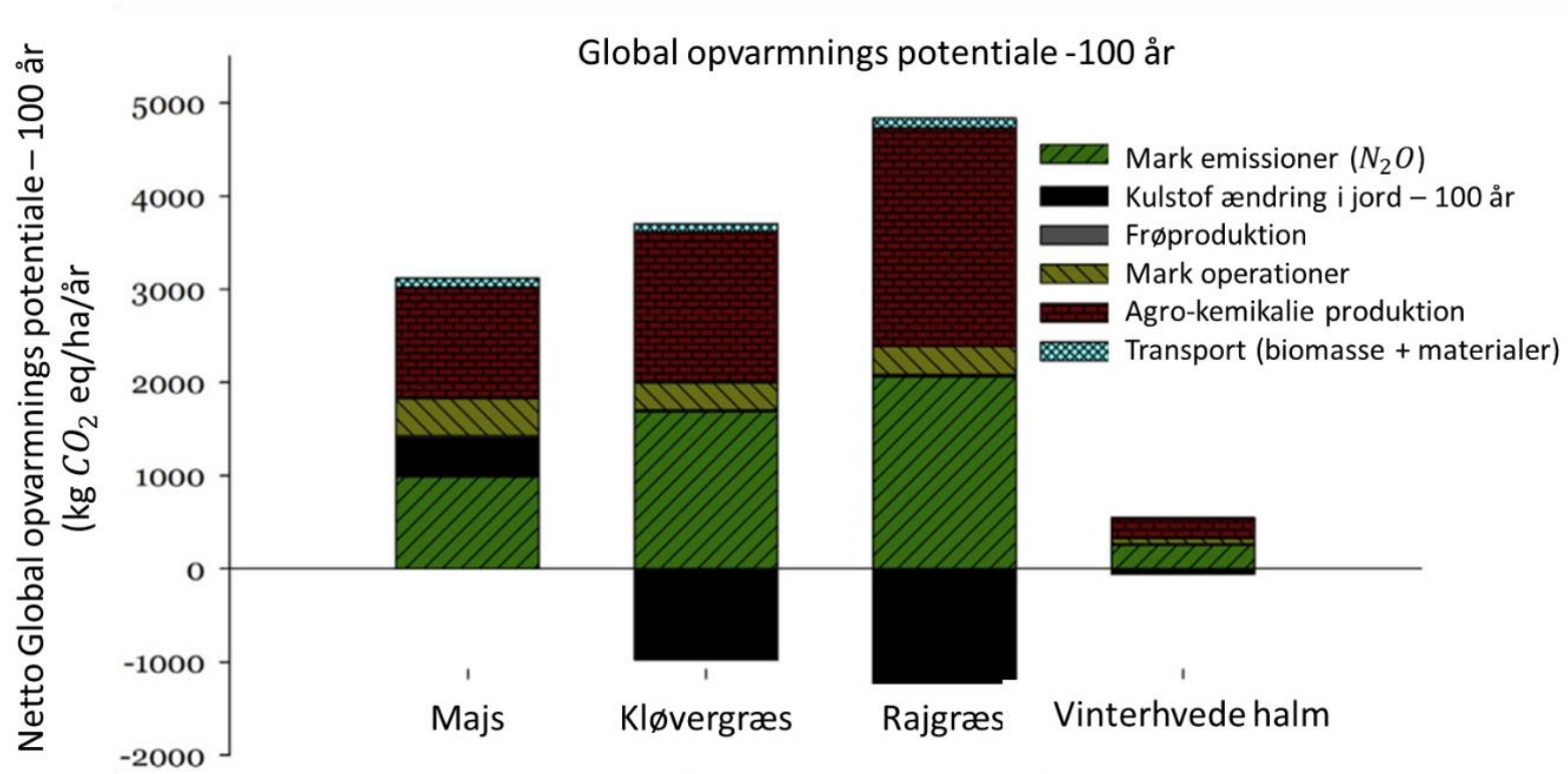
Figur 2, global opvarmnings potentiale ved produktion af konventionel majs, kløvergræs, rajgræs og halm. Produktionskædens emissioner er medtaget. Modificeret efter (Parajuli et al., 2017).
